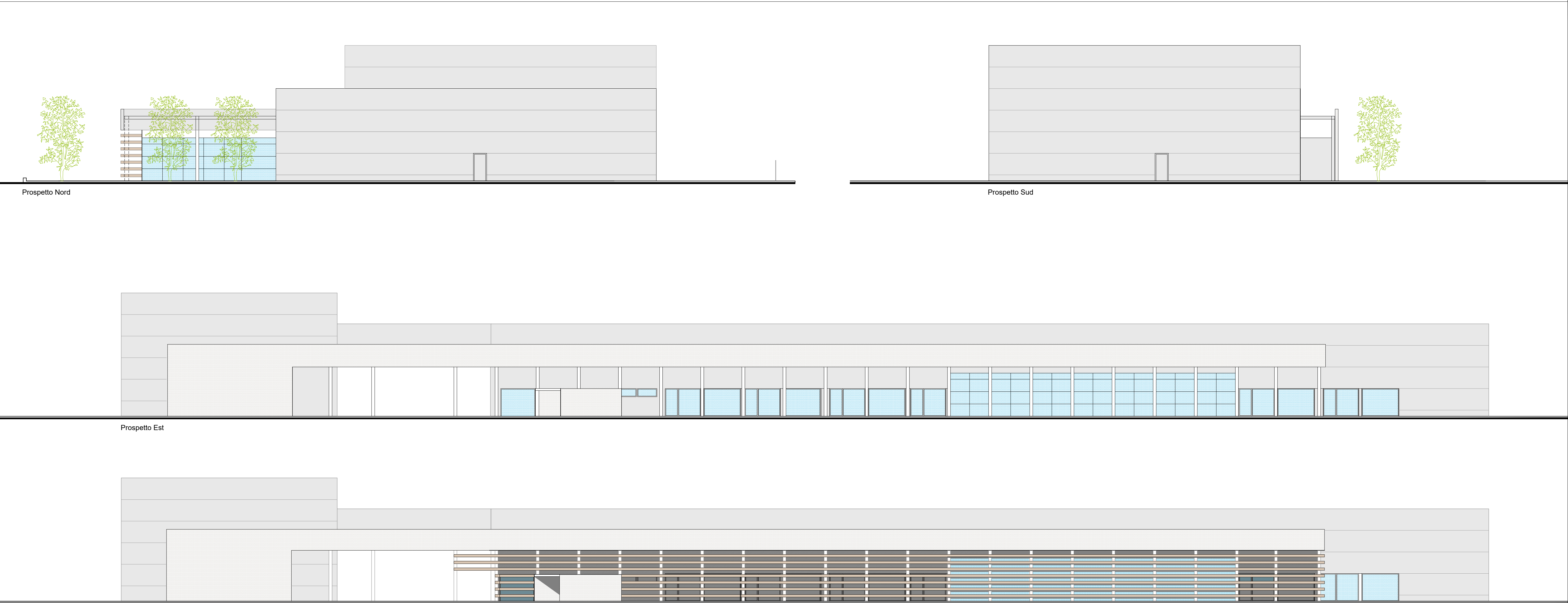
PROSPETTI scala 1:200
